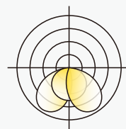
双偏光 (100x90x15°)
